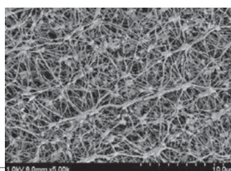
メンブレンの組織 電子顕微鏡・5,000倍拡大写真
